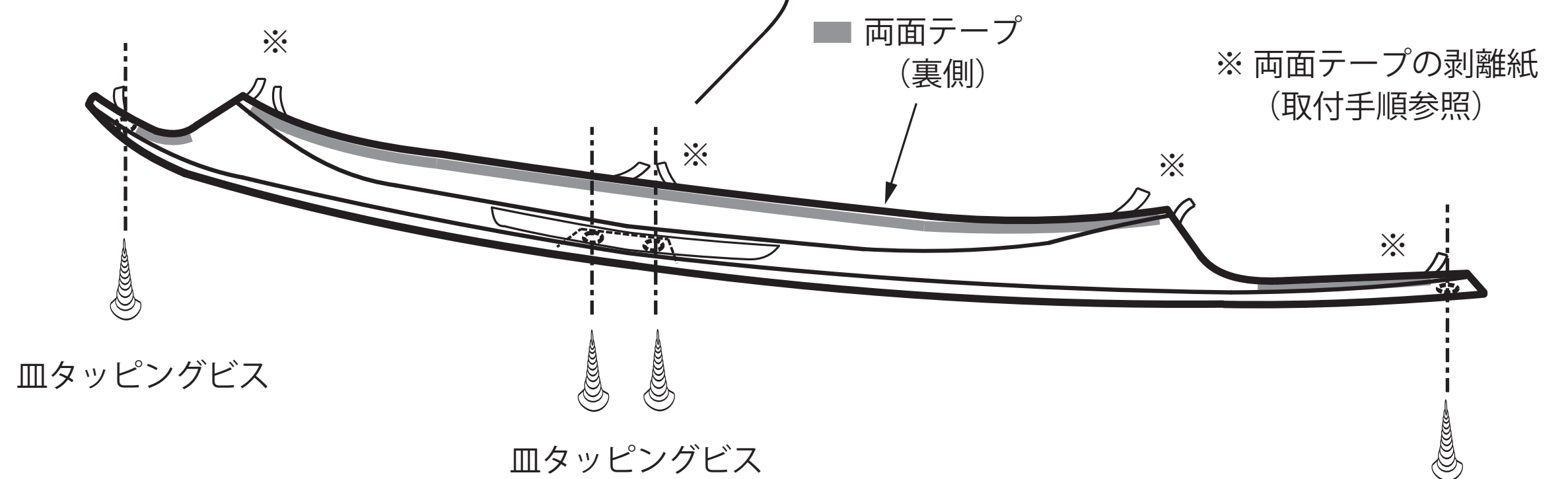
フロントリップスポイラー
